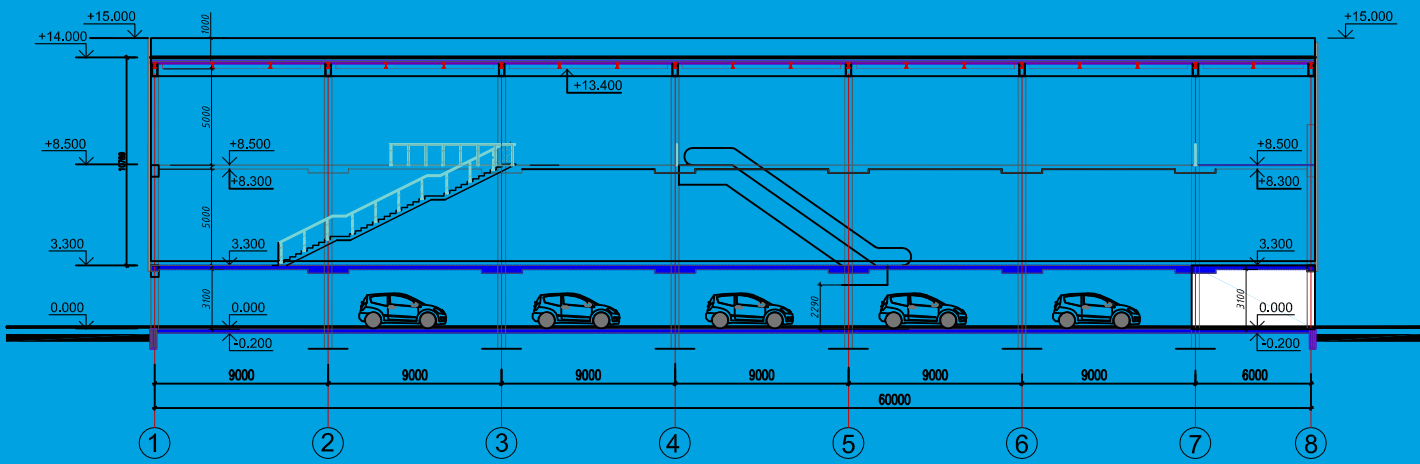
Разрез 1-1
